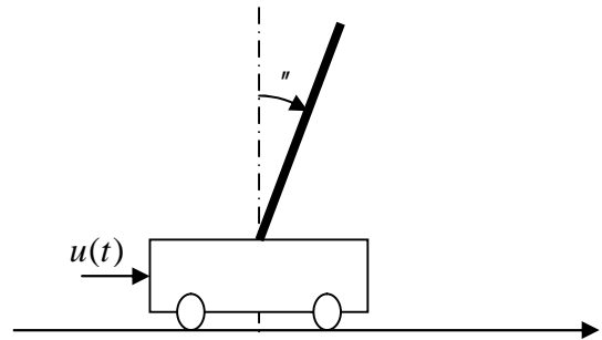
Fig.2. Schéma de principe du pendule inversé
